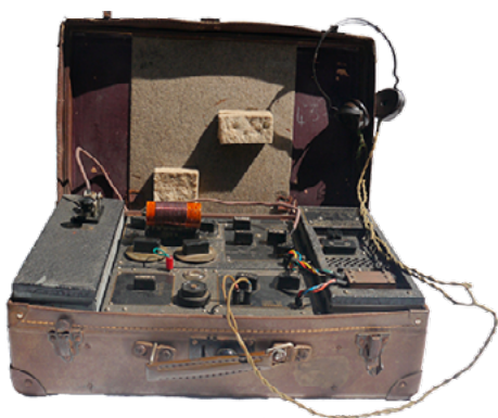
Valise émetteur- récepteur ondes courtes. AAMRN/collection historique, 1985
